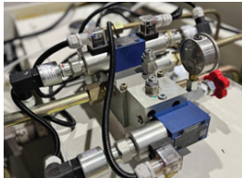
Bloco hidráulico de segurança c/ válvulas monitoradas Sistema de segurança frontal Laser multi-feixes
