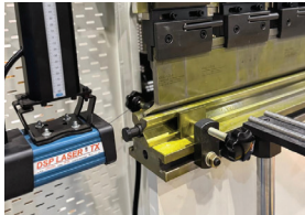
Bloco hidráulico de segurança c/ válvulas monitoradas Sistema de segurança frontal Laser multi-feixes
