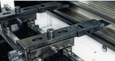
Encosto traseiro com guias lineares e fuso de esferas Servo-acionado
